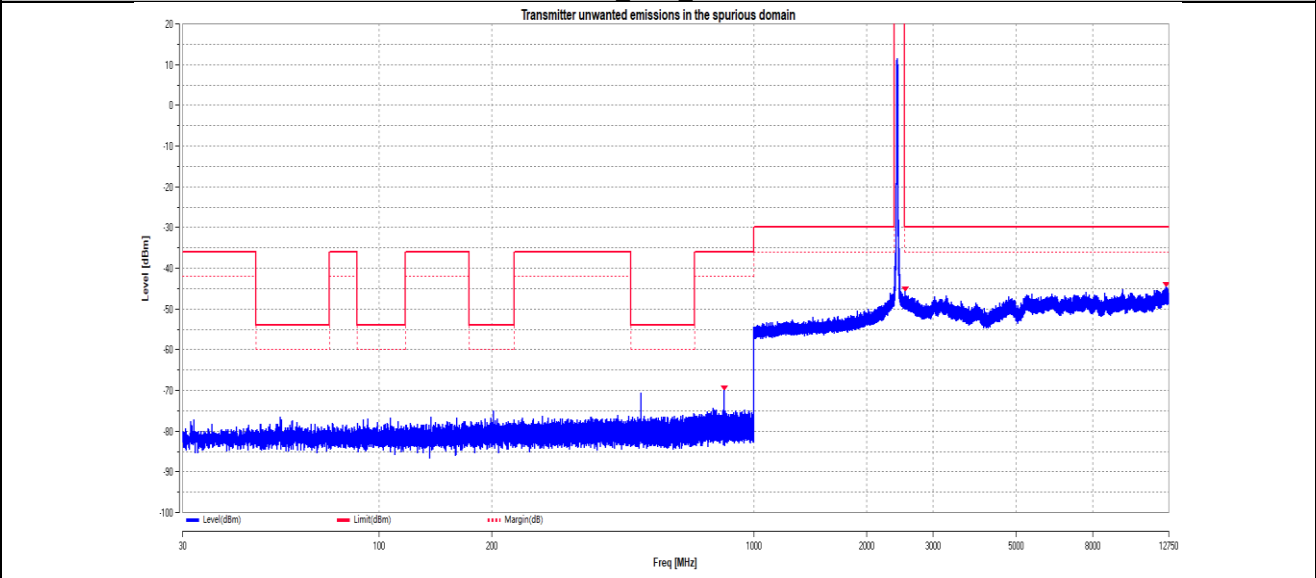
11G Ant1 2472
