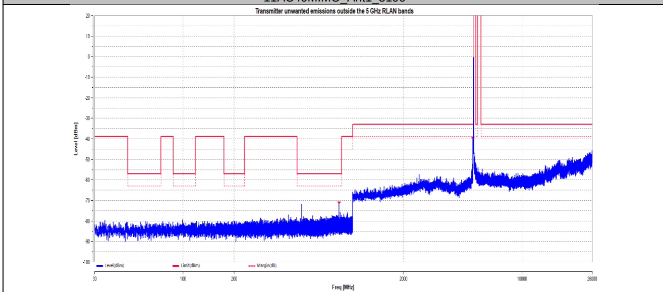
11AC40MIMO_Ant2_5190
