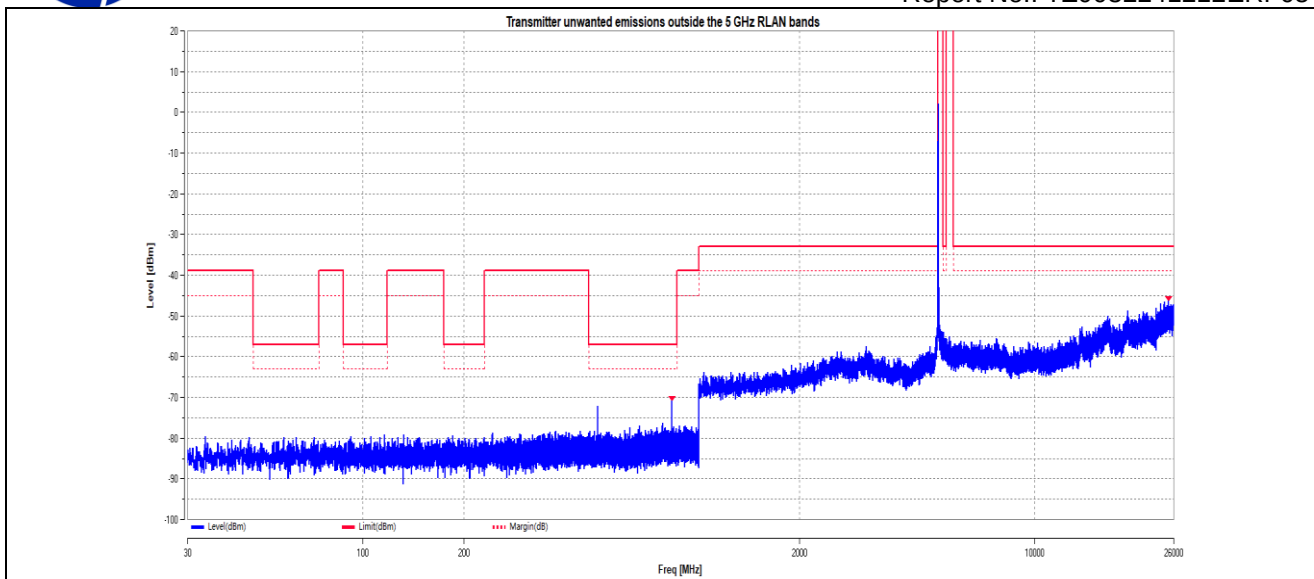
11AC20MIMO_Ant2_5180
