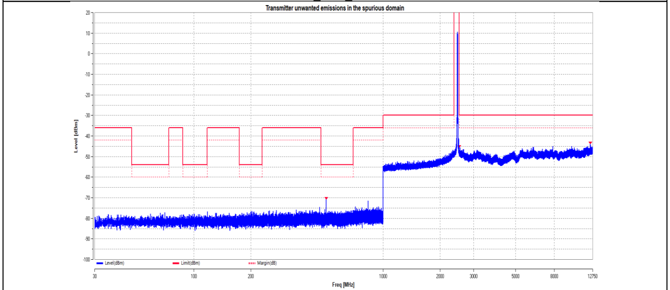
11N20MIMO Ant1 2412
