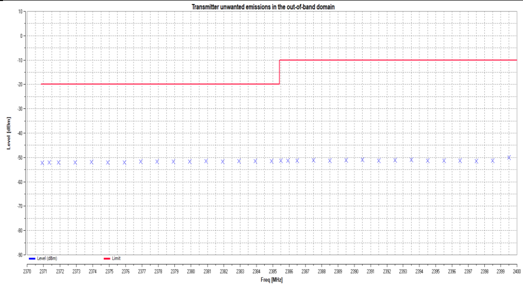
11B_Ant2 2472 2483.5MHz to 2483.5MHz+2BW
