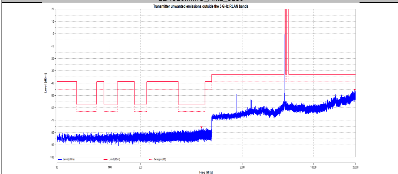
11AC40MIMO_Ant1_5190
