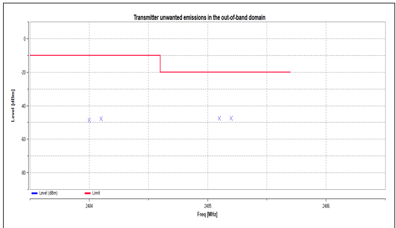
(OOB_BLE_1Mbps_2480MHz)
