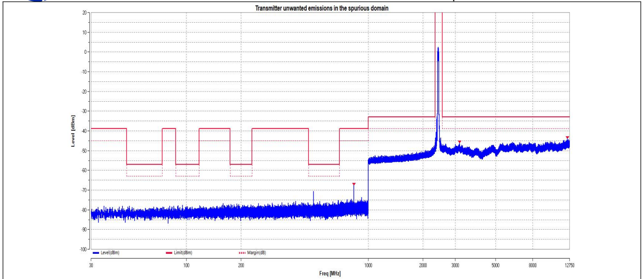
11N40MIMO_Ant2_2422
