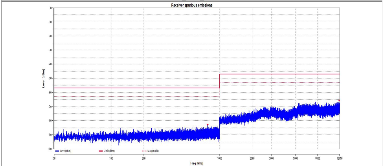
3DH5 Ant1 2480
