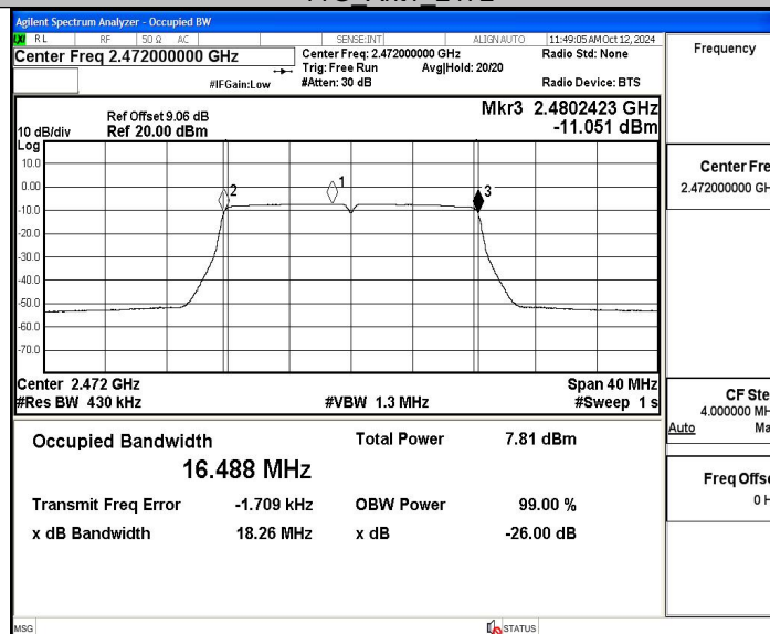
11G_Ant2_2472
