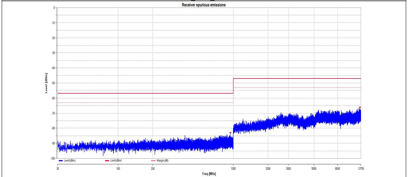
11G_Ant2_2412
