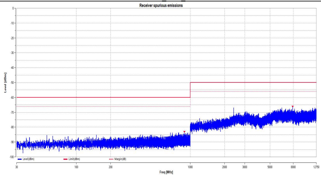
11N40MIMO_Ant2_2462
