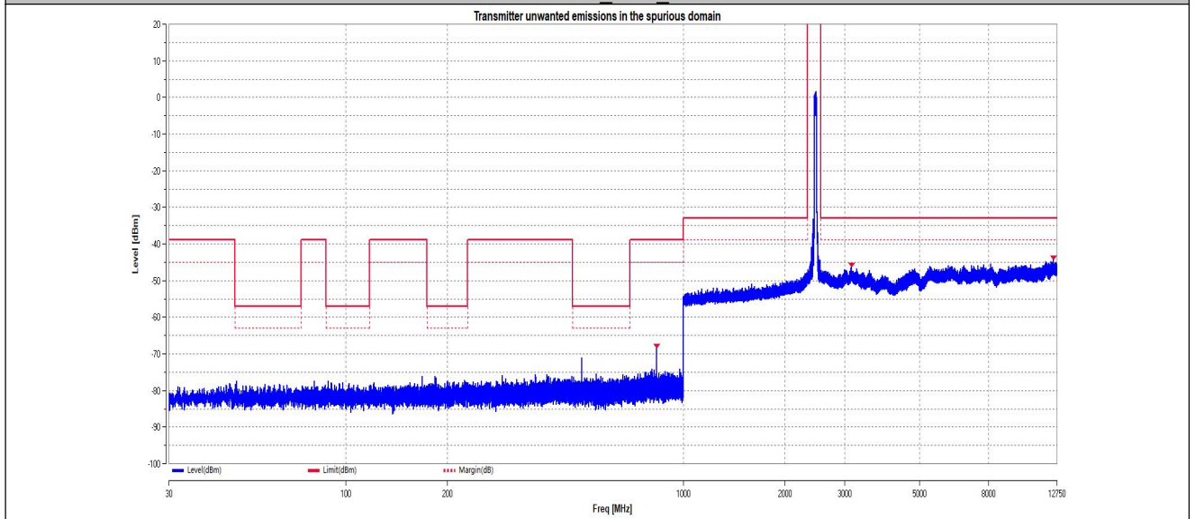
11N40MIMO_Ant2_2462
