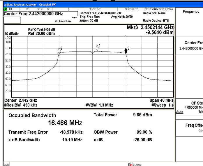
11G_Ant1_2472
