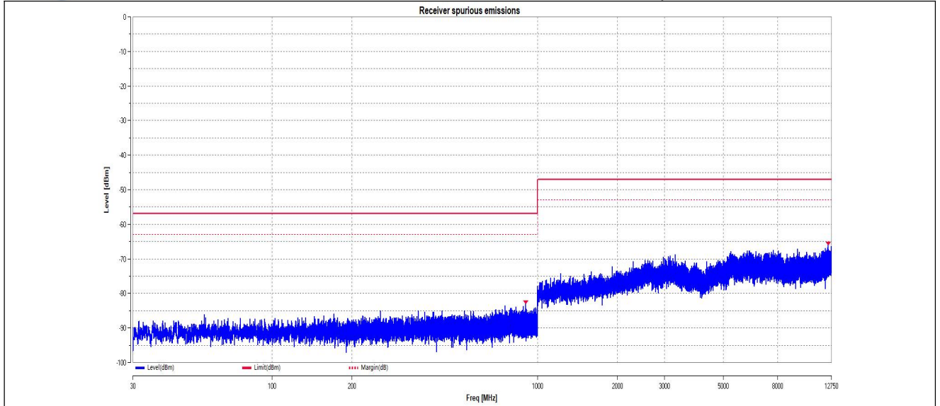
2DH5 Ant1 2480
