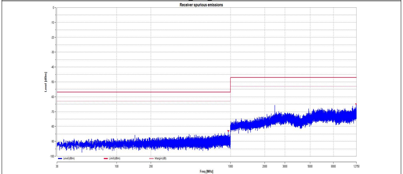
11N20MIMO Ant1 2412
