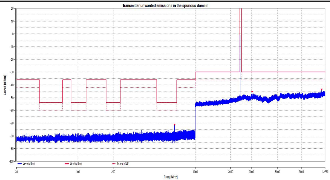
3DH5 Ant1 2480
