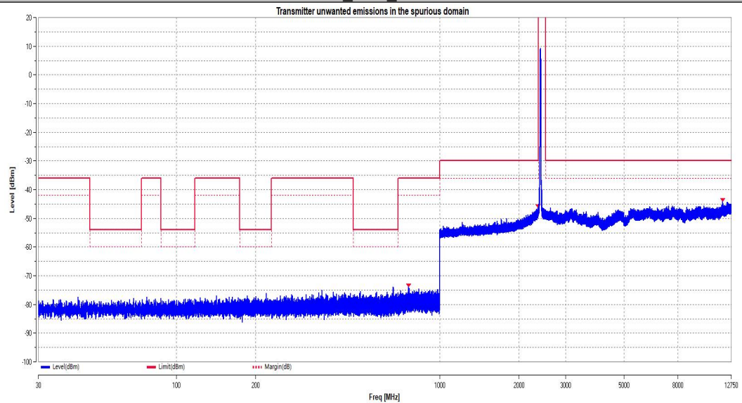
11G_Ant2_2412
