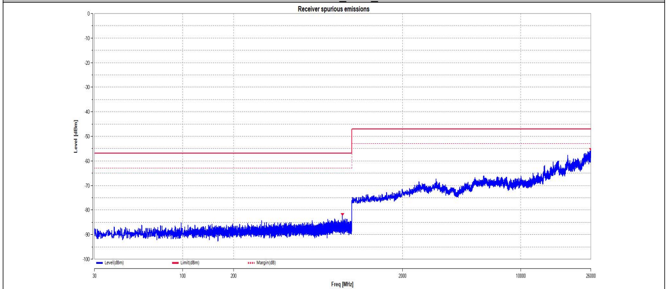
11AC80MIMO_Ant2_5210
