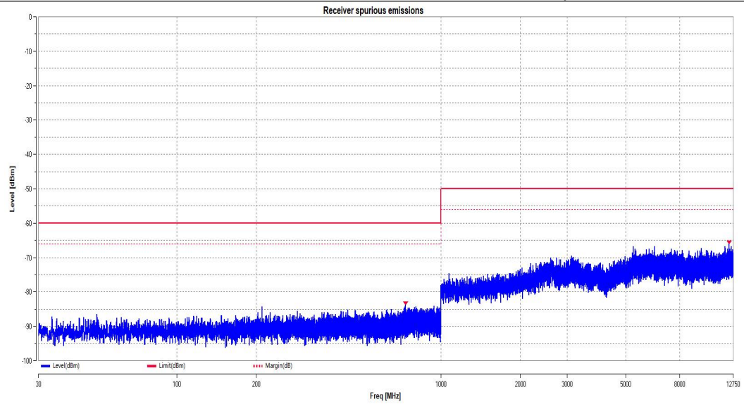
11N40MIMO_Ant2_2422
