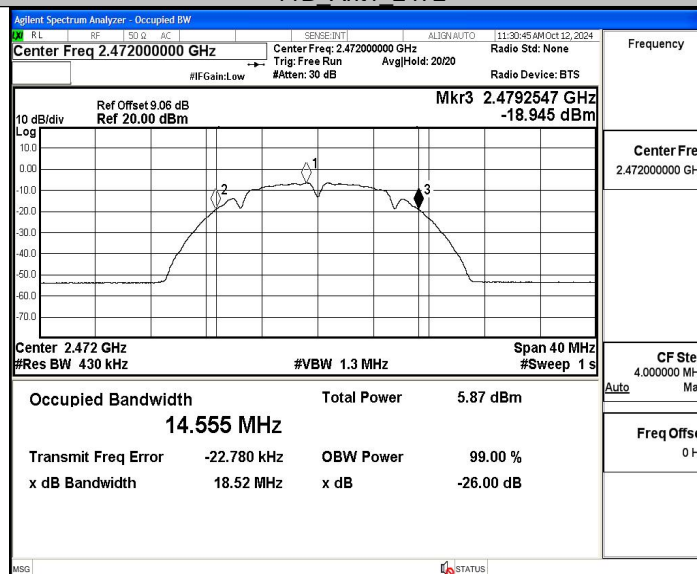
11B_Ant2_2472
