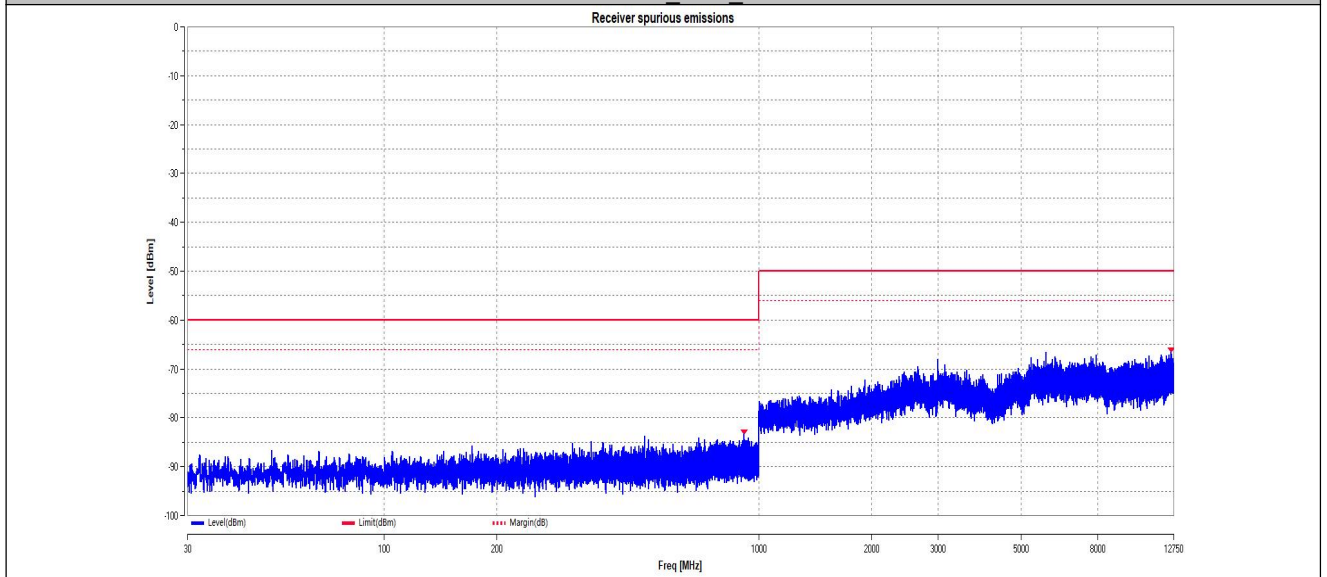
11N40MIMO_Ant1_2422
