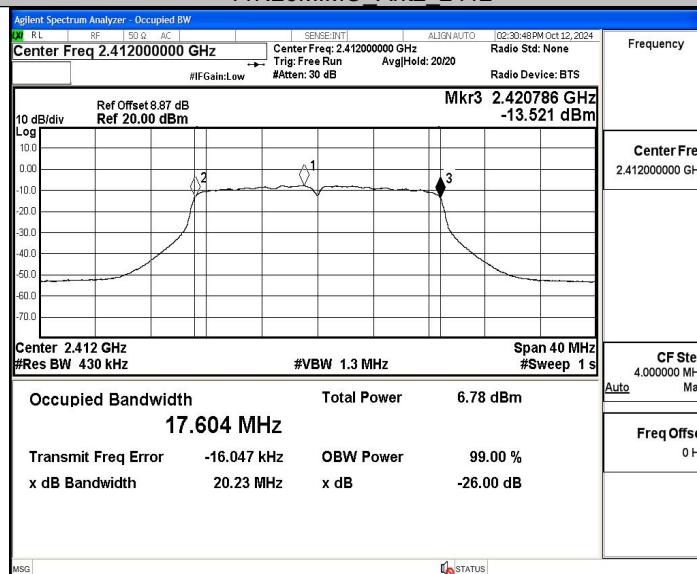
11N20MIMO_Ant1_2442
