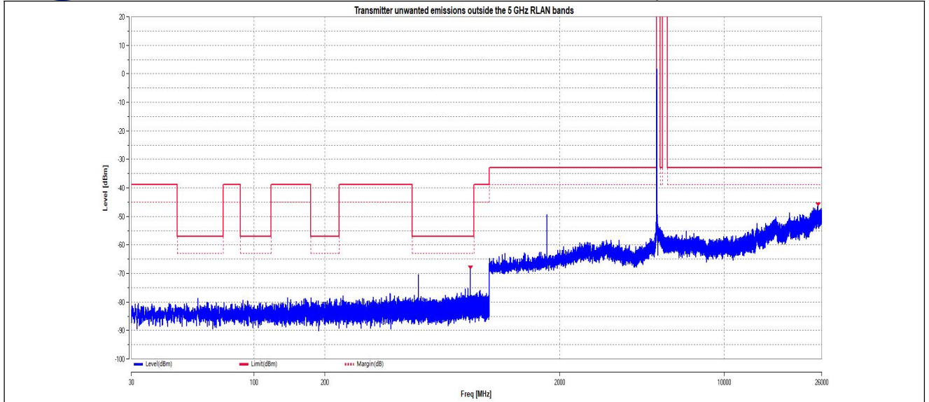
11AC20MIMO_Ant2_5180
