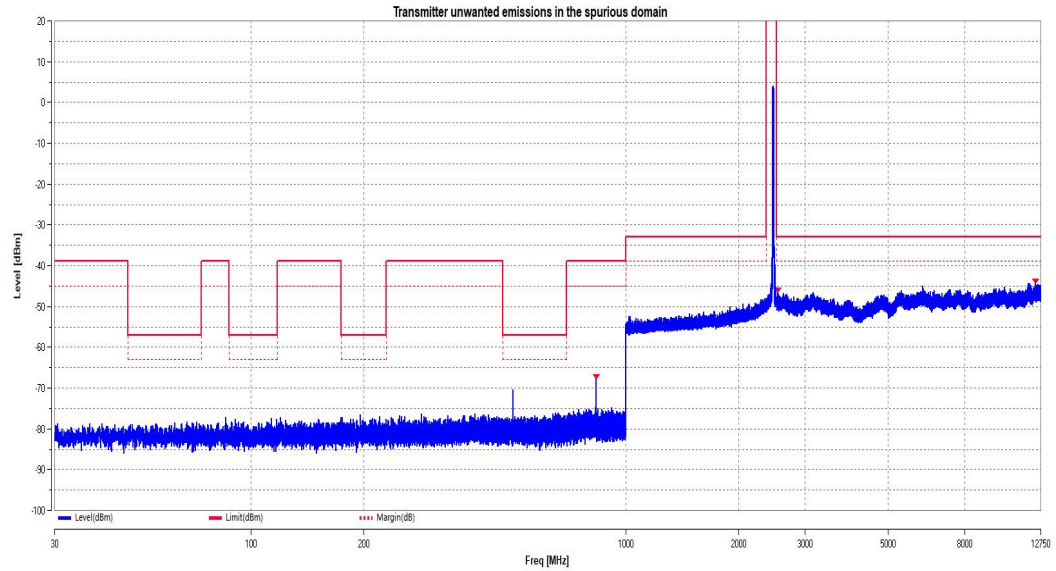
11N20MIMO_Ant2_2472
