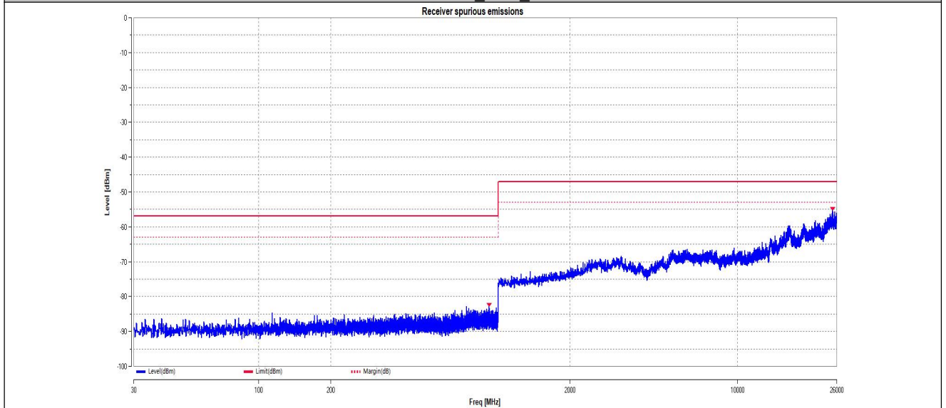
11N40MIMO_Ant2_5190
