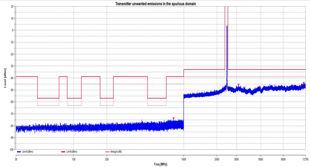
11N40MIMO_Ant1_2422
