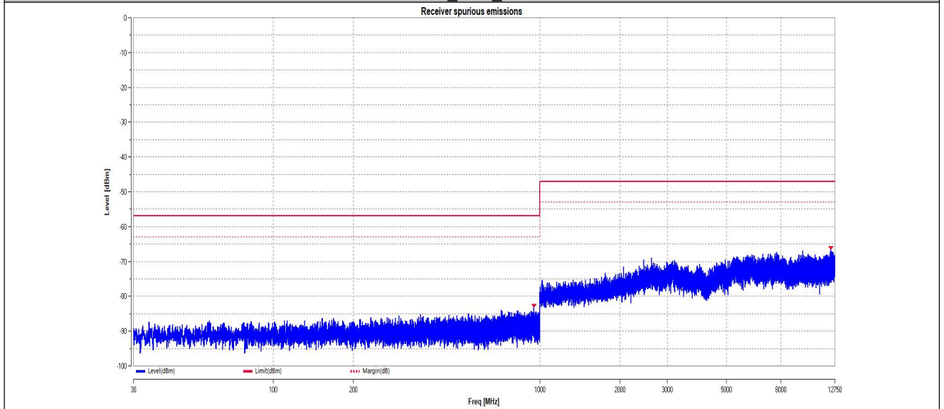
3DH5 Ant1 2402
