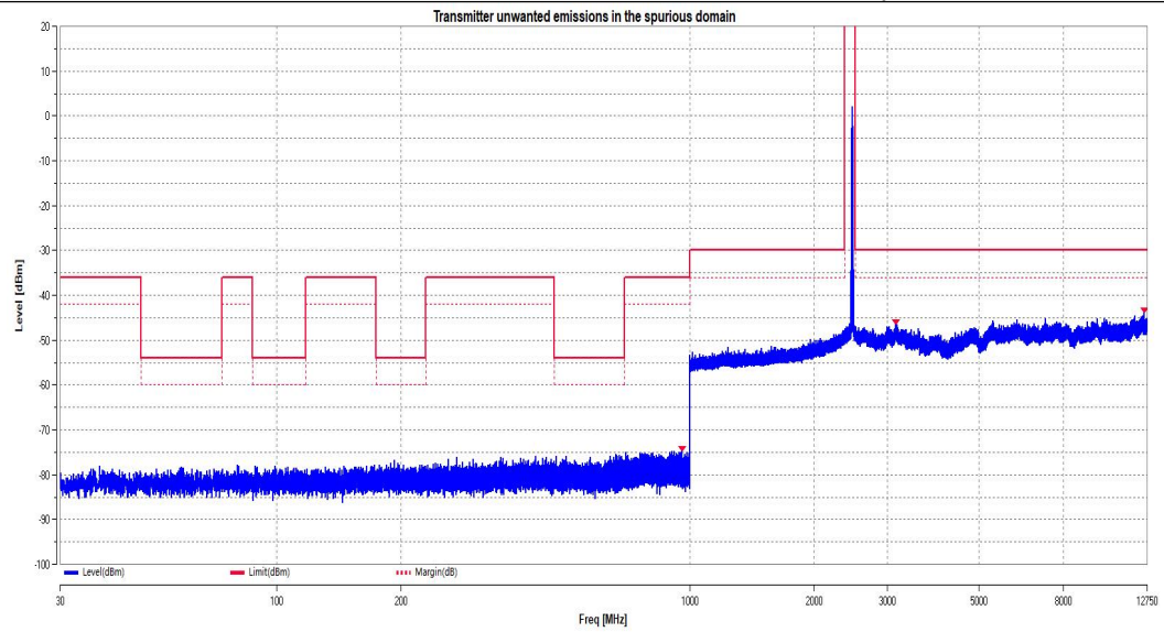
11G_Ant1_2412
