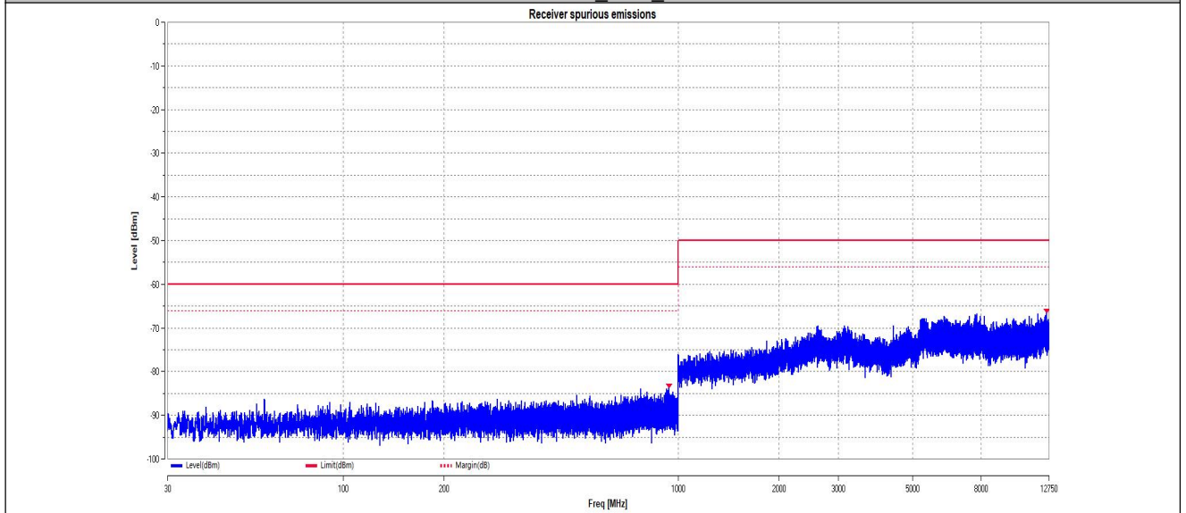
11N20MIMO_Ant2_2472
