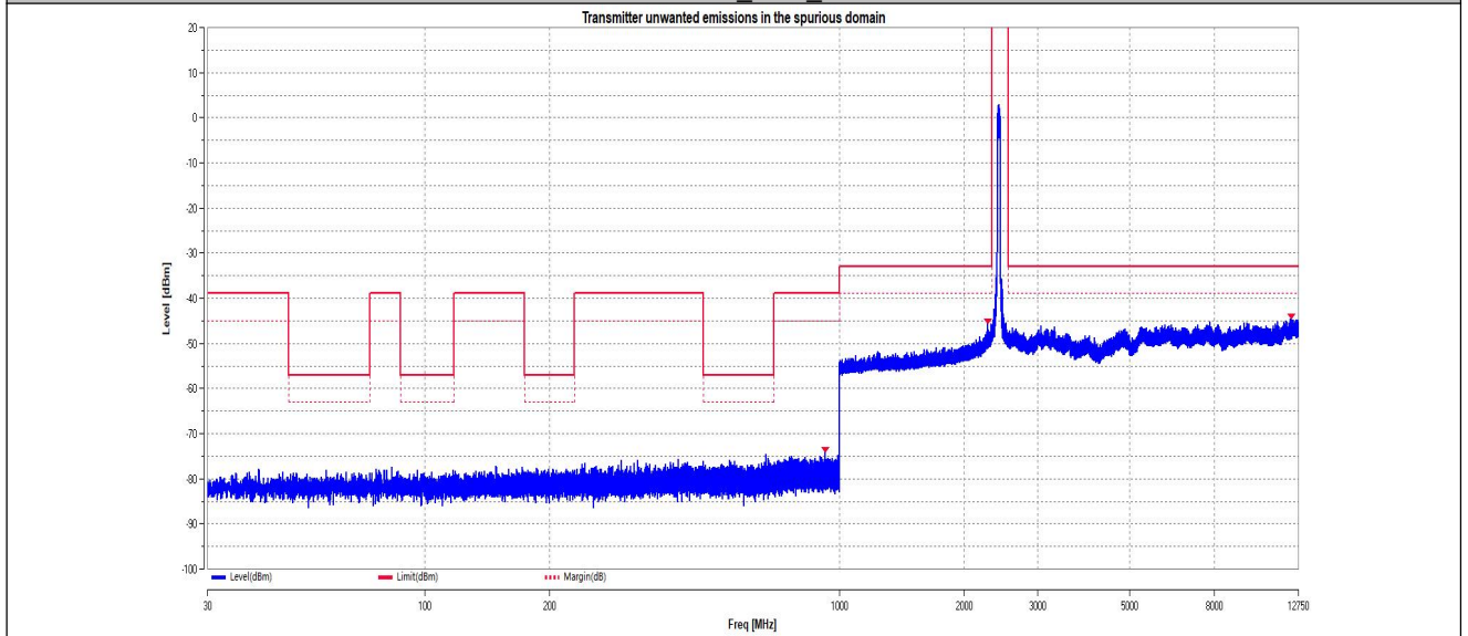
11N40MIMO_Ant1_2462
