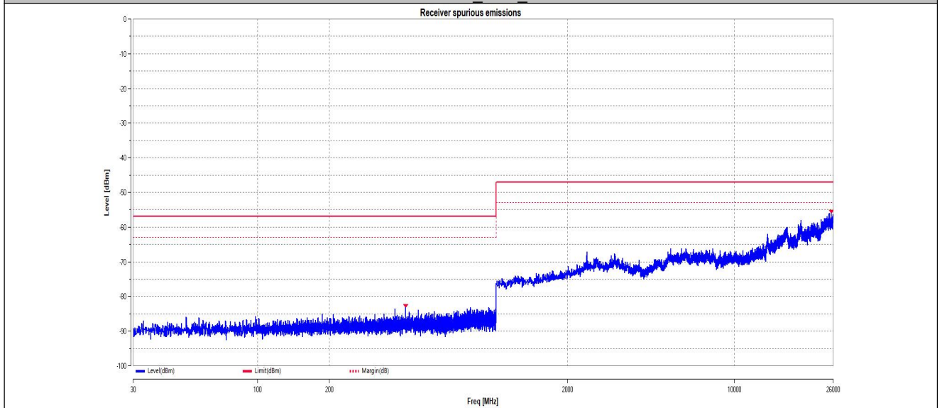
11AC20MIMO_Ant1_5180
