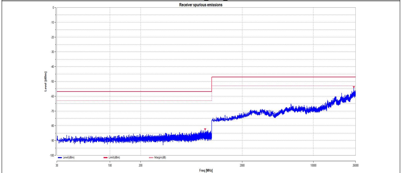
11AC80MIMO_Ant2_5210
