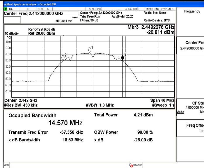
11B_Ant2_2442
