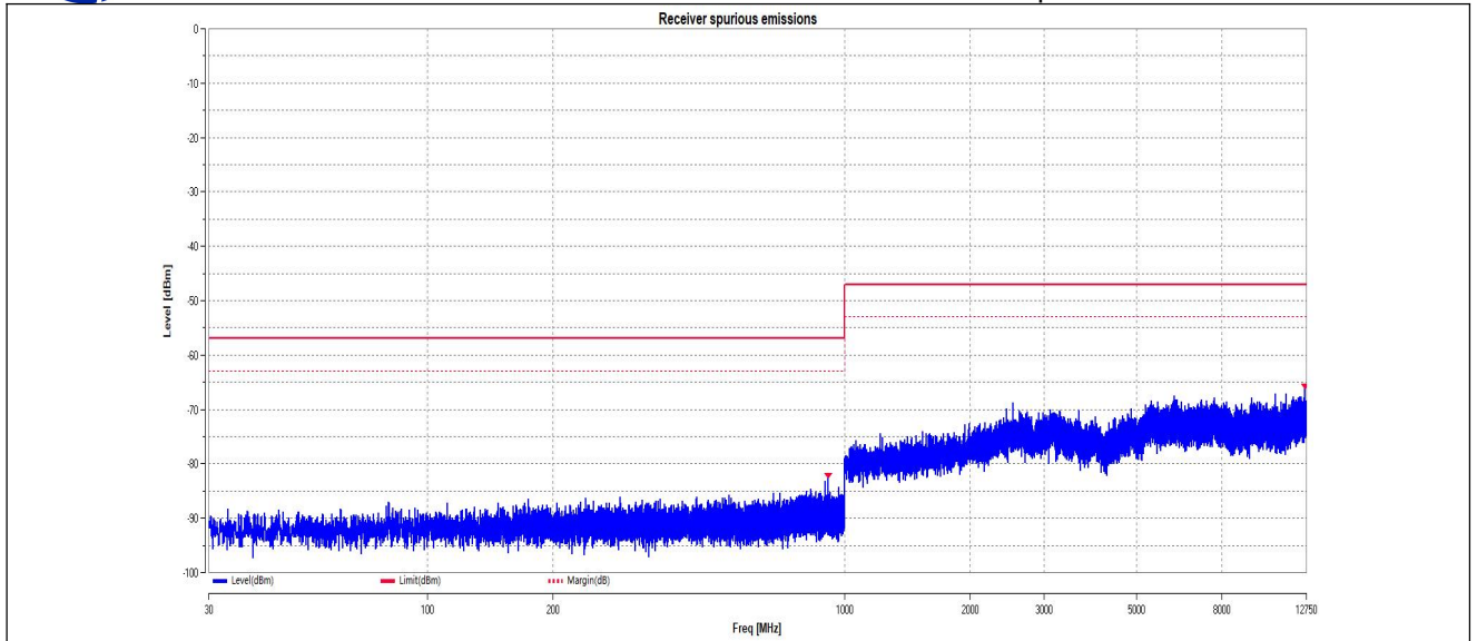
11G_Ant1_2412
