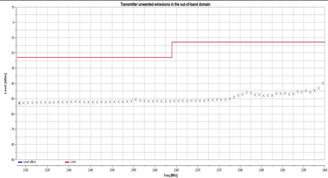
11N40MIMO_Ant1_2422_2483.5MHz+2BW
