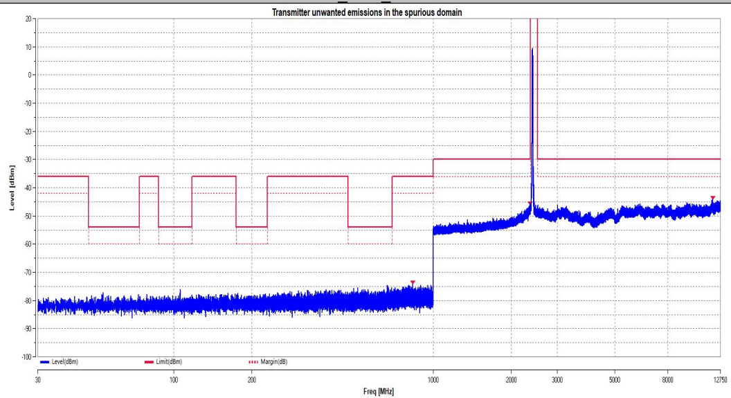
11G_Ant1_2472
