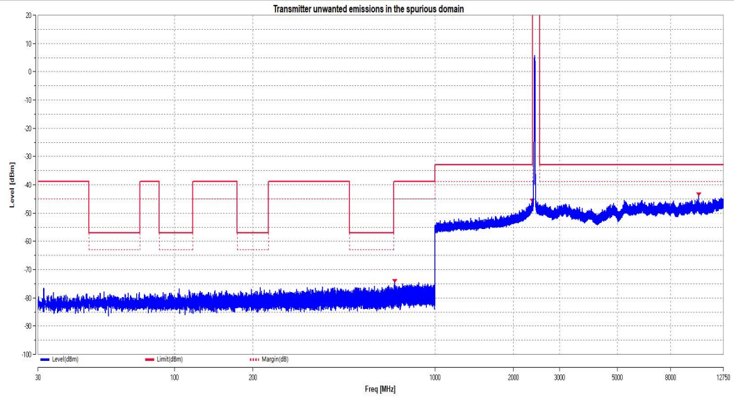
11N20MIMO_Ant1_2472
