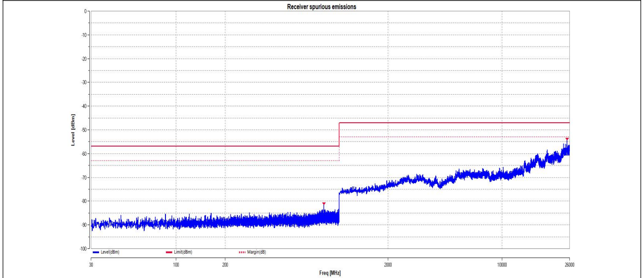
11AC40MIMO_Ant1_5190
