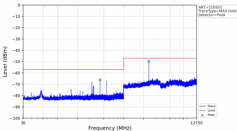
802.11b_2412MHz_Ant1 (SISO)_NTNV
