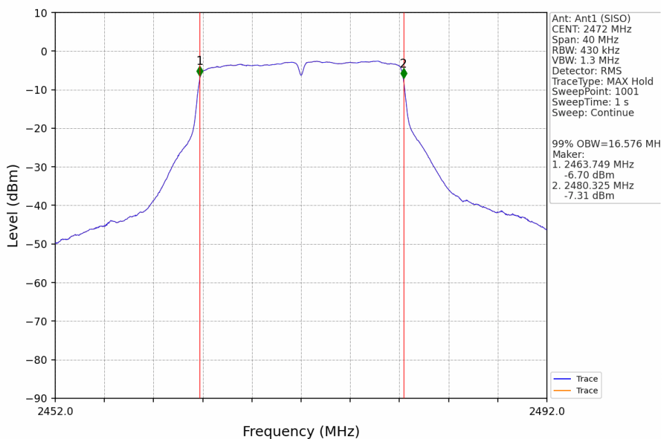
802.11g_2472MHz_Ant1 (SISO)_NTNV
