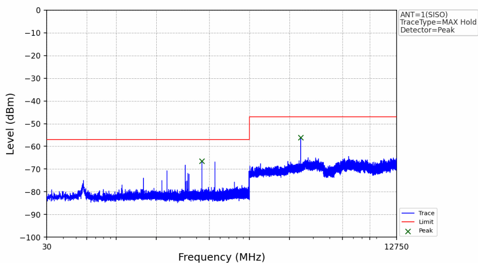
802.11b_2472MHz_Ant1 (SISO)_NTNV
