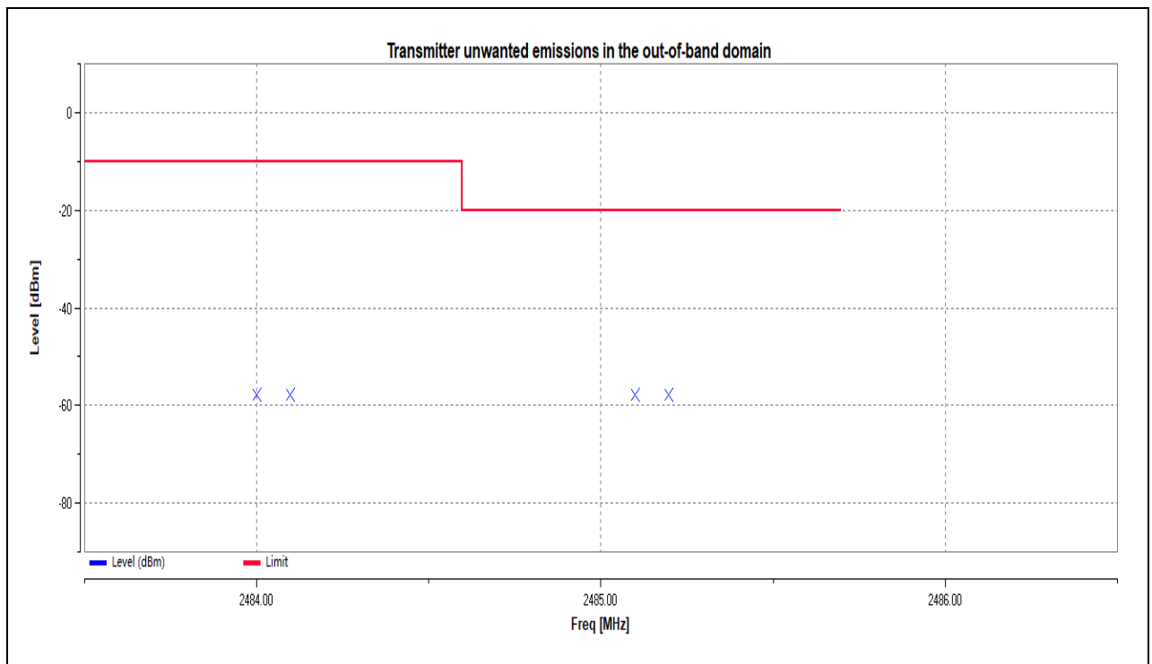
(OOB_BLE_1Mbps_2480MHz)
