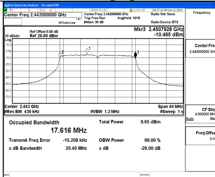
11N20SISO_Ant1_2472
