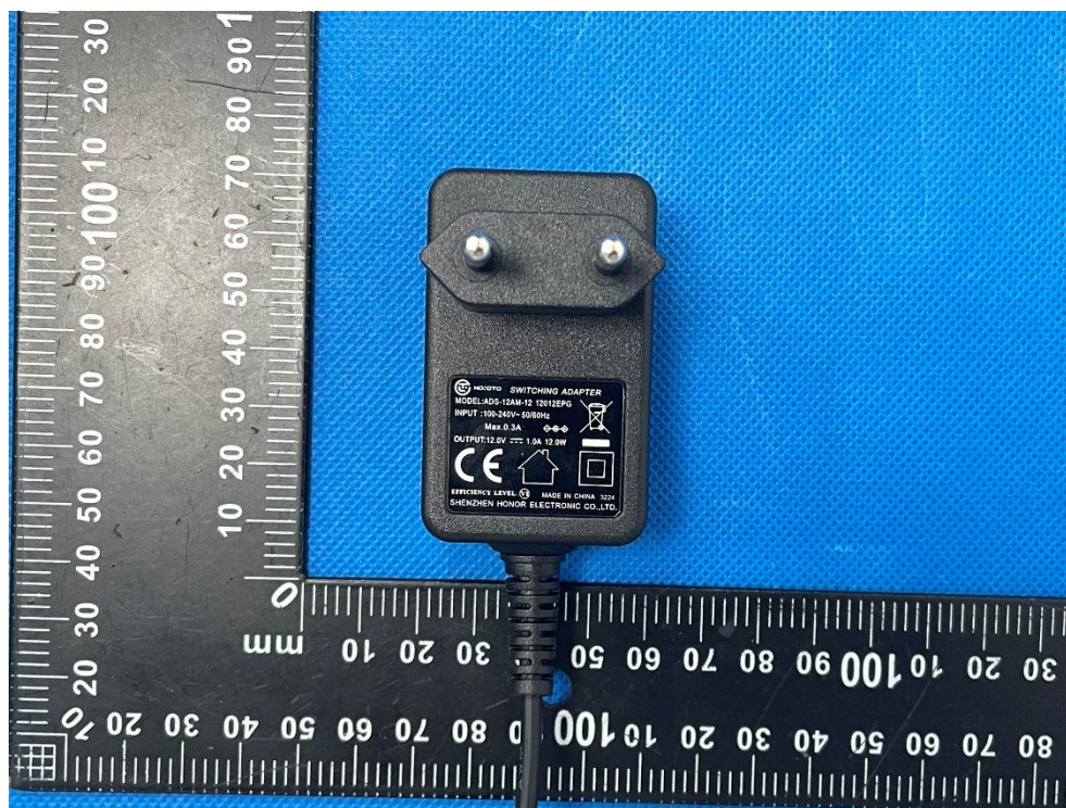
EUT PHOTO 17
