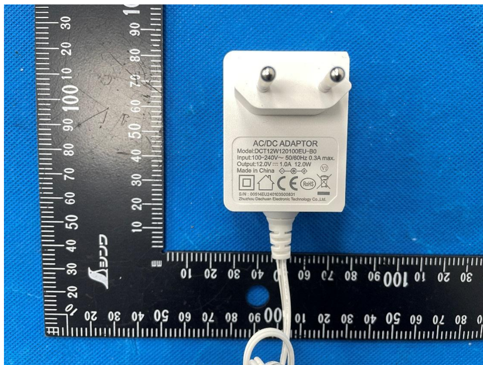
EUT PHOTO 18
