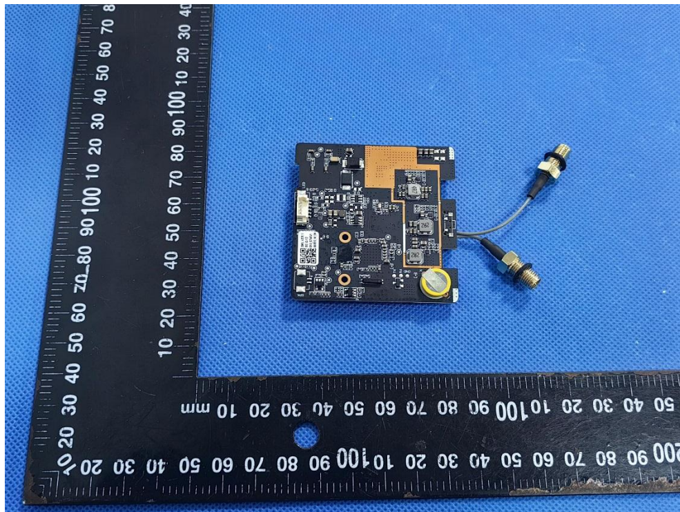
EUT PHOTO 13
