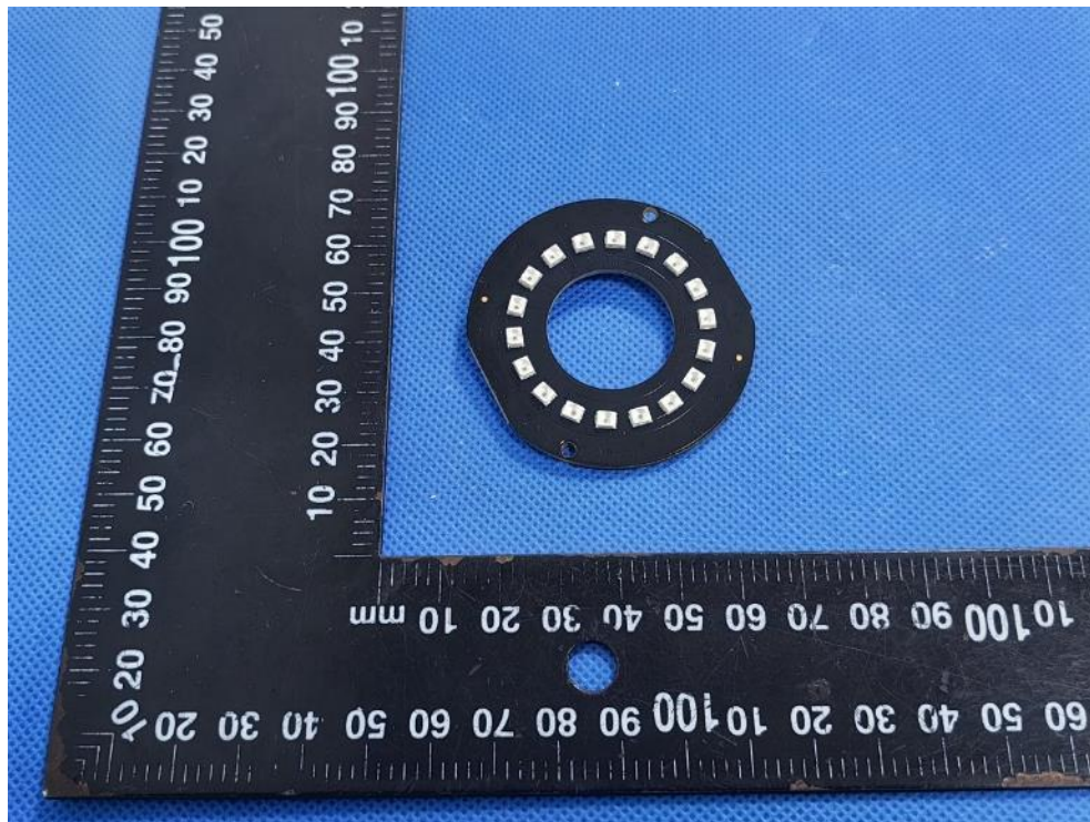
EUT PHOTO 11
